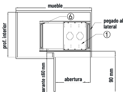
MUEBLE CON PARANTE
